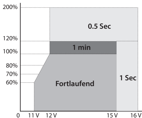
Leistung vs. Ausgangsspannung
