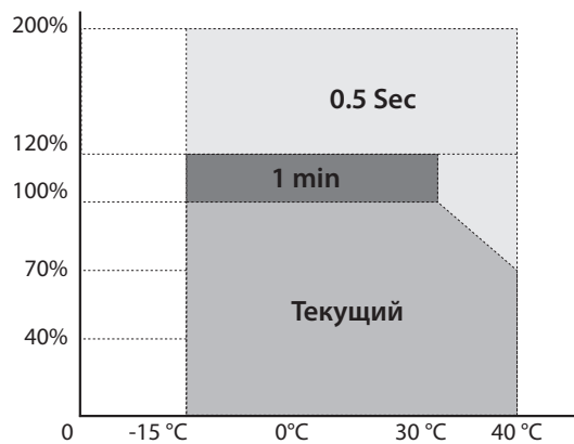
Мощность как функция температуры
